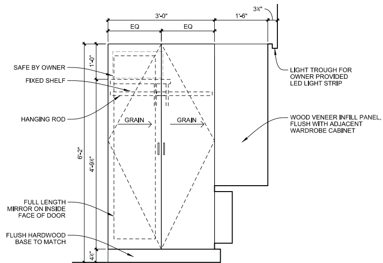
ELEVATION B
