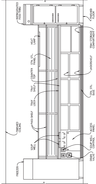
7 ELEVATION
