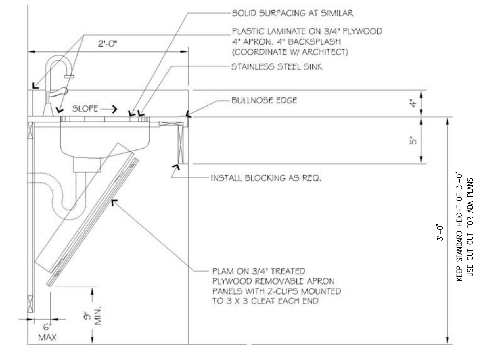
ADA CABINET SIDE VIEW N.T.S.
