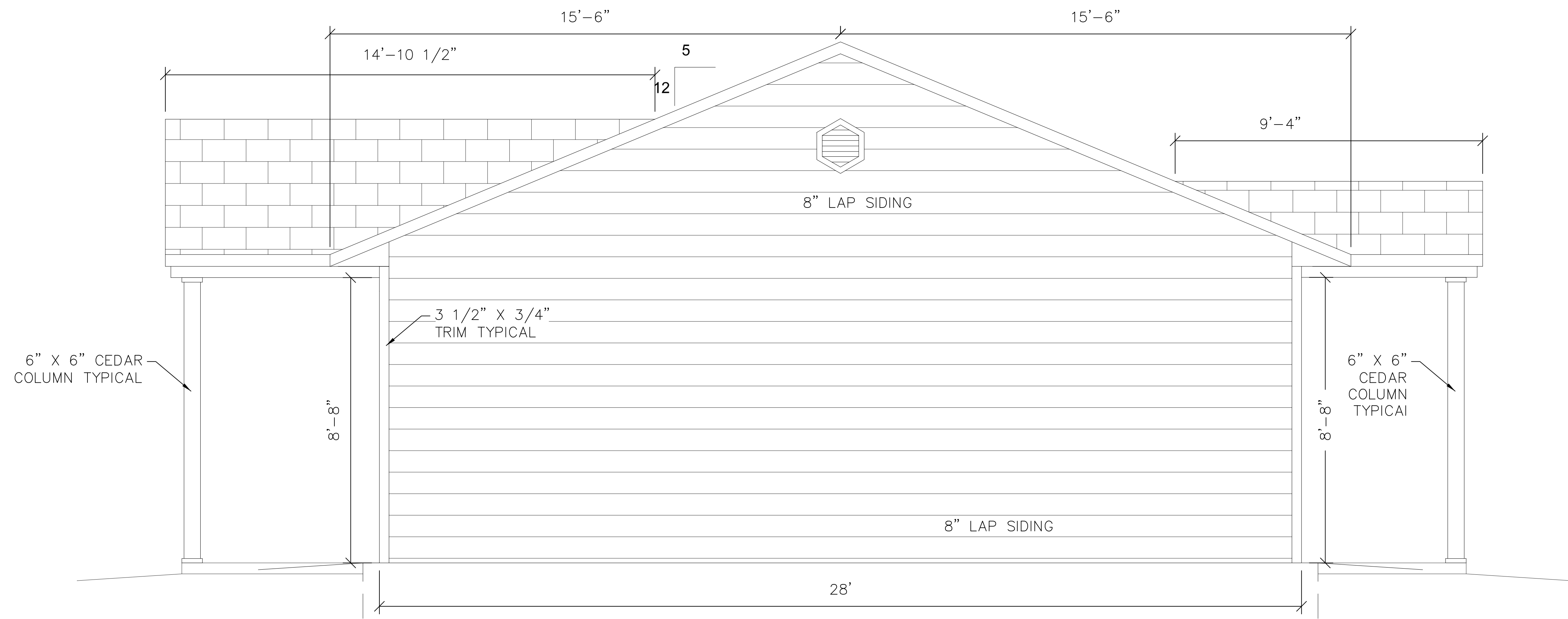
RIGHT ELEVATION
