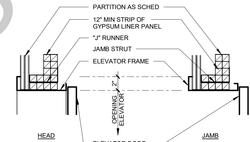
ELEVATOR DOOR DETAIL DRYWALL 1 1/2\"/>
