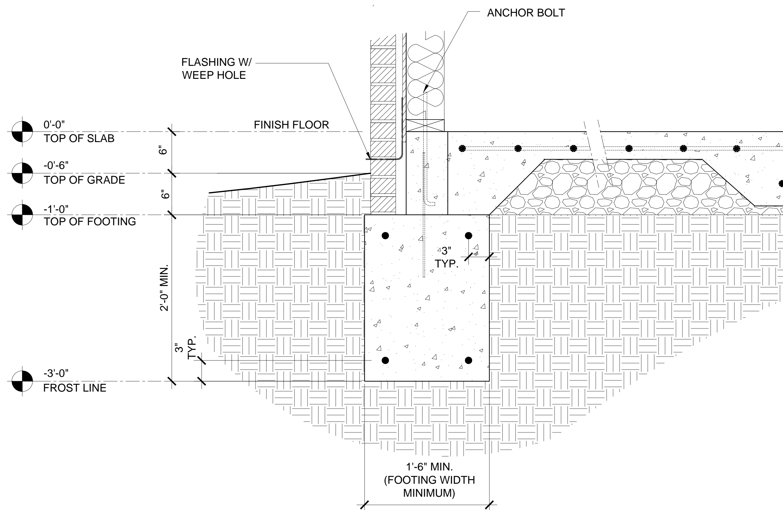
2 DETAIL SCALE: 1 1/2" = 1'-0"
