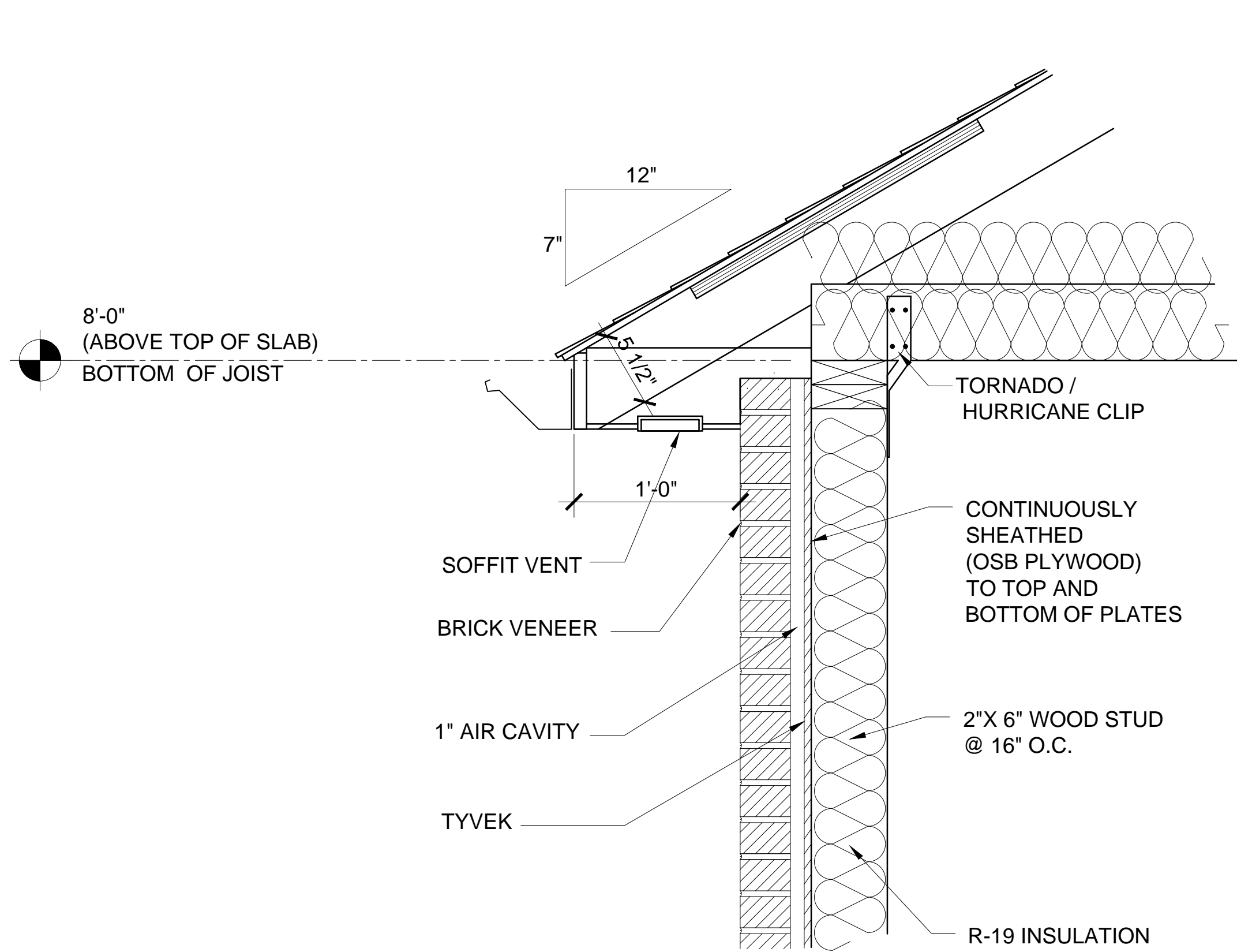
3 DETAIL SCALE: 1 1/2" = 1'-0"
