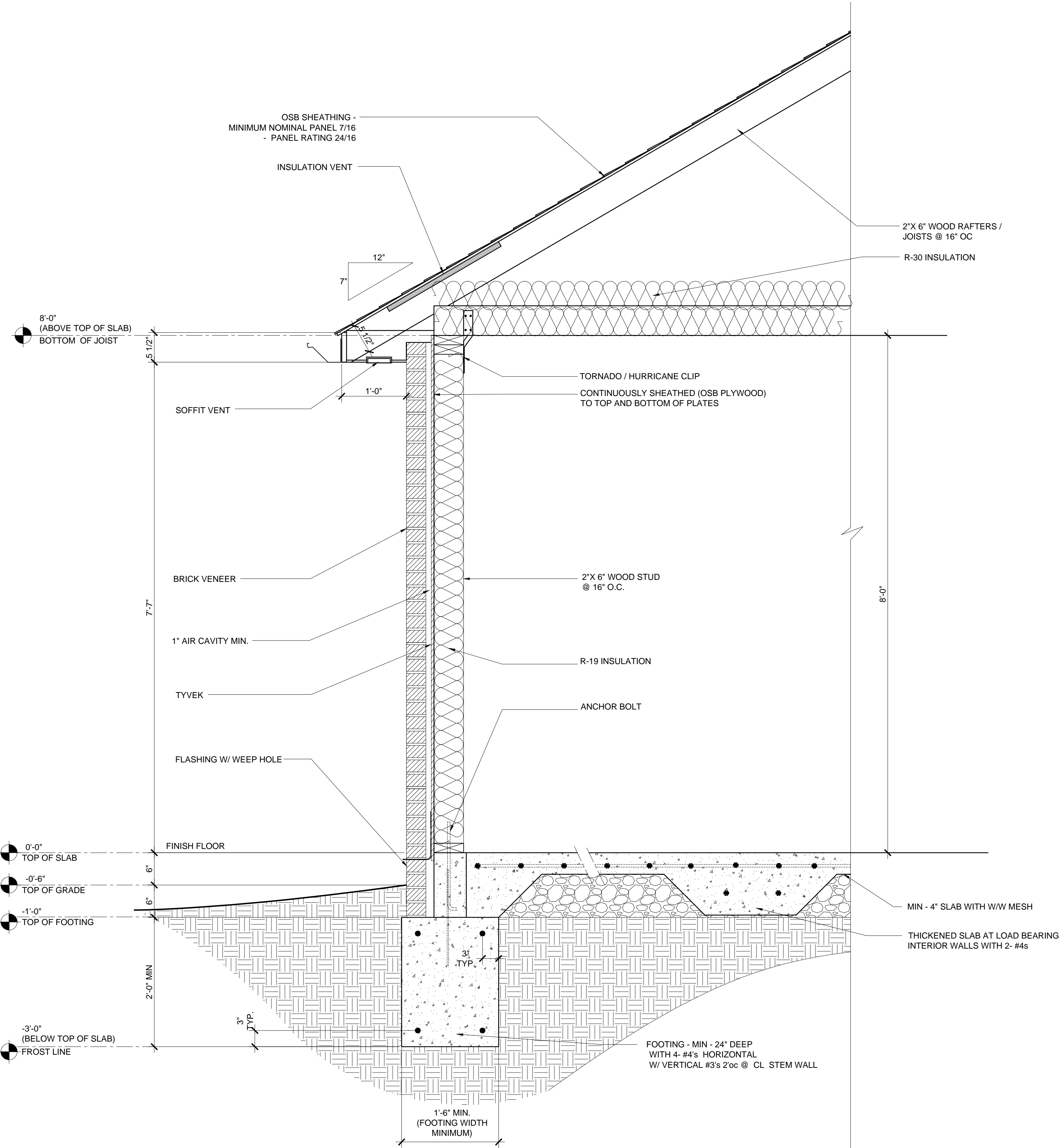
1 SECTION - EXTERIOR WALL SCALE: 1" = 1'-0"
