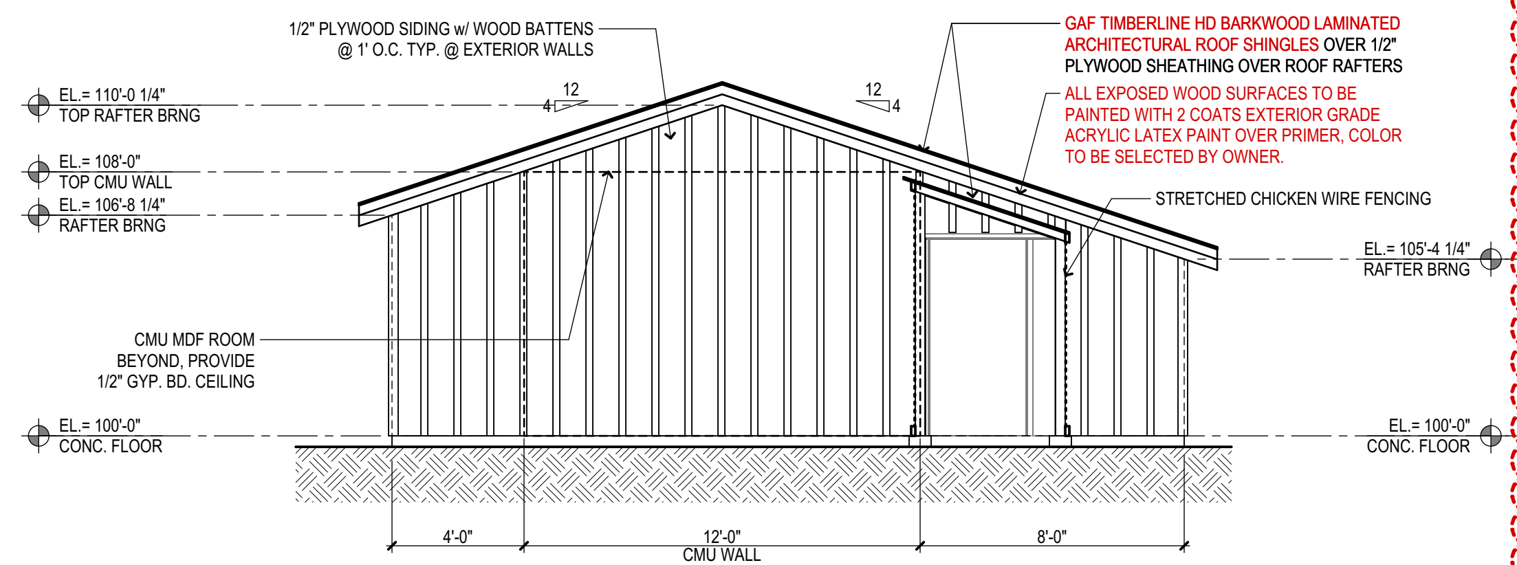
4 ELEVATION
