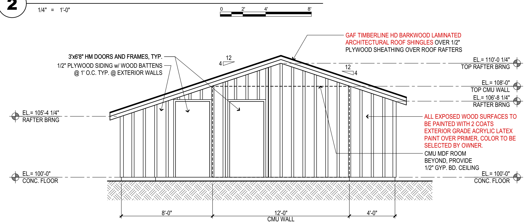
1 ELEVATION
