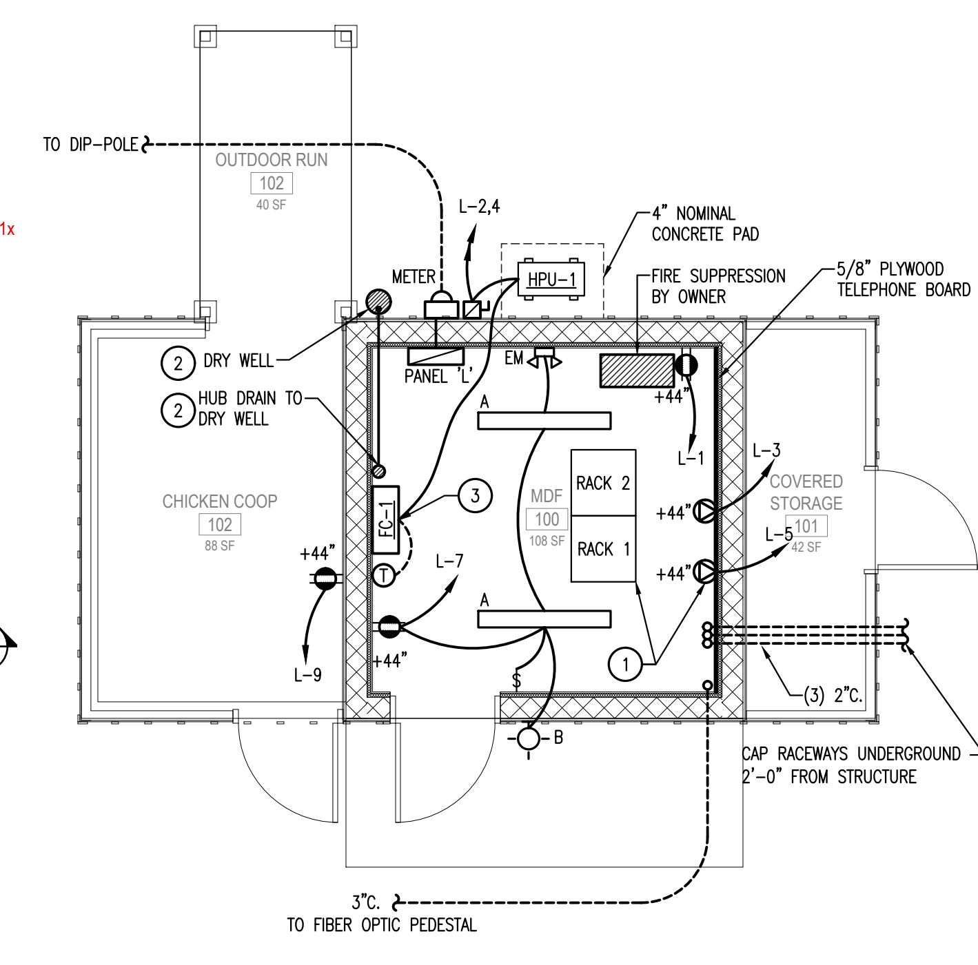
6 MEP PLAN
