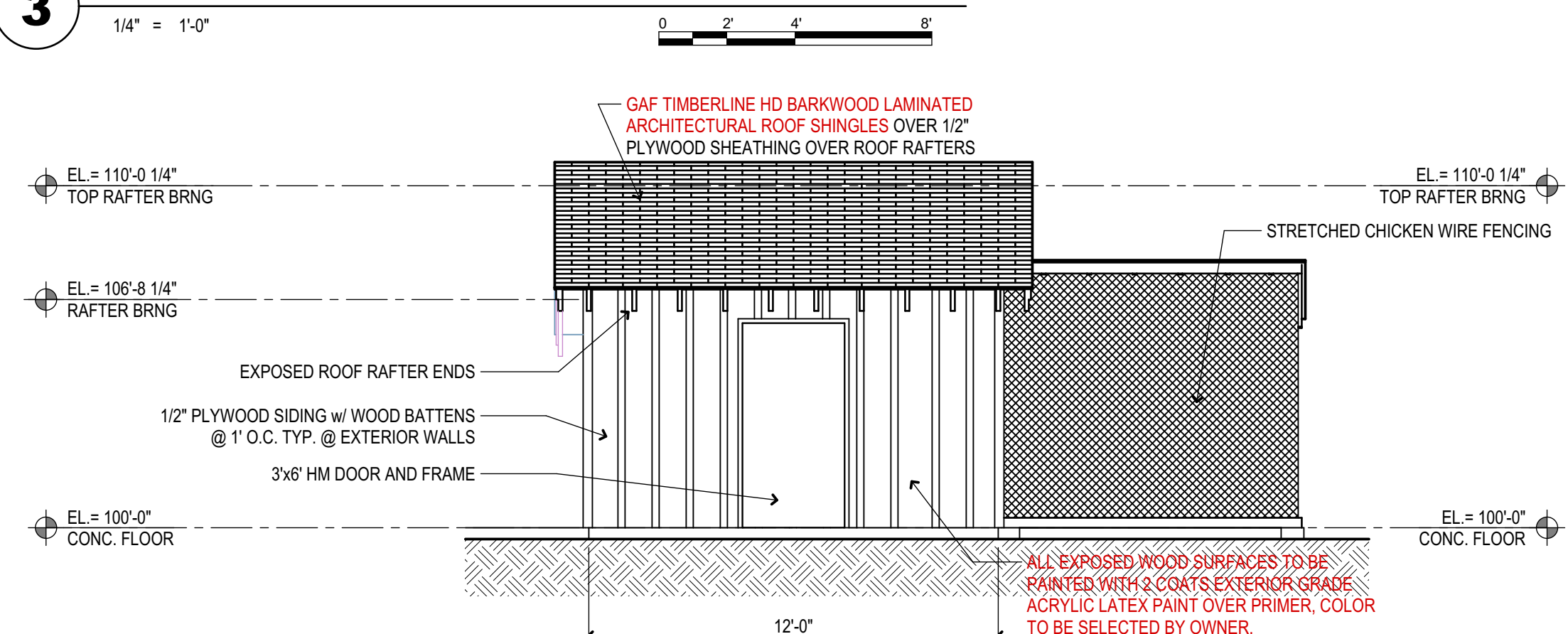
2 ELEVATION
